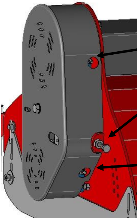
Tension galet accessible
